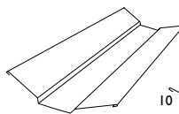
Ендова внешняя Общая длина 2000 мм Эффективная длина 1900 мм
