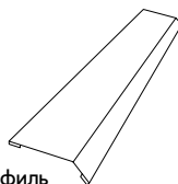
Карнизный профиль Общая длина 2000 мм Эффективная длина 1900 мм
